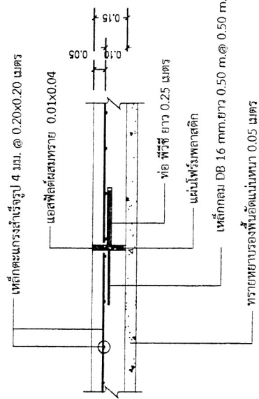
ขยาย EXPANSION JOINT scale ทุกระยะ 50 เมตร 1:20
