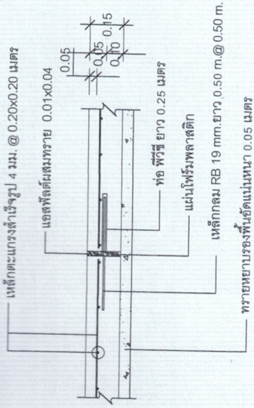
ขยาย EXPANSION JOINT scale 50 เมตร 1:20
